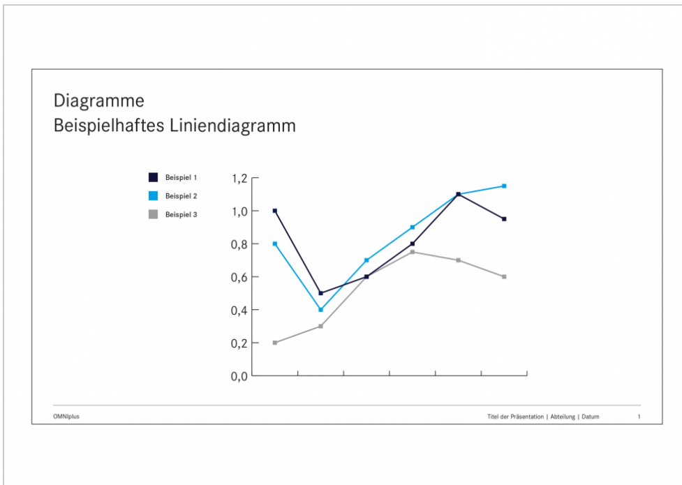
Beispielhaftes Liniendiagramm
